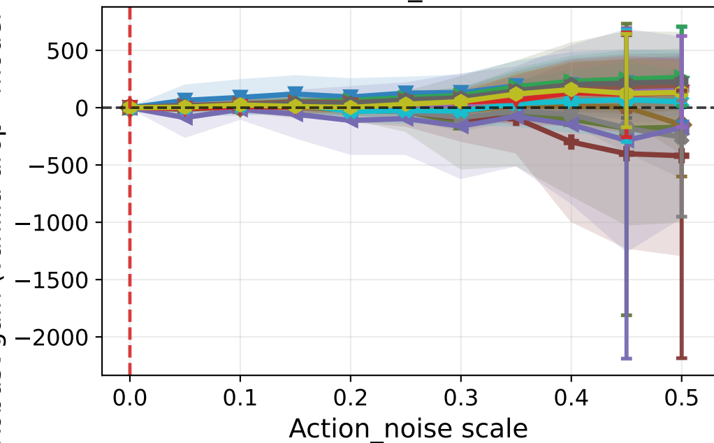
Action_noise
